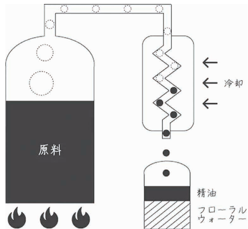
アロマオイルの抽出工程
